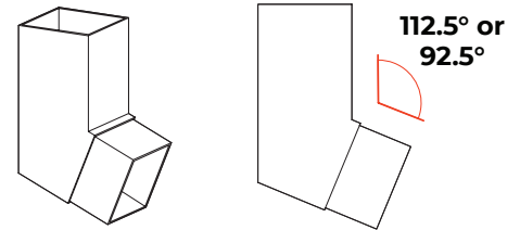
112.5° bend shown
