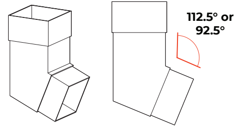
112.5° bend shown
